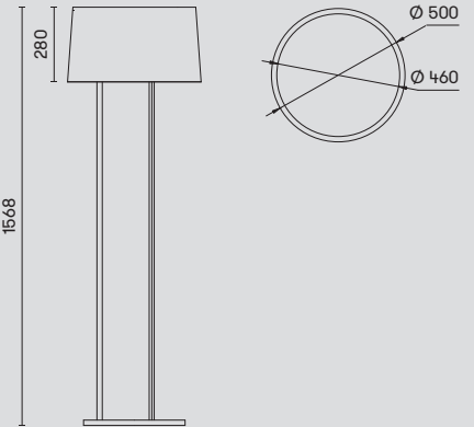
Top diffuser | Difusor Superior | Diffuseur Supérieur
