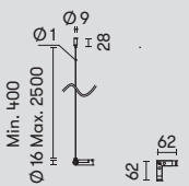
71-8259-05-05 ■ 90° horizontal connector | Conector 90° horizontal | Connecteur 90° horizontal
