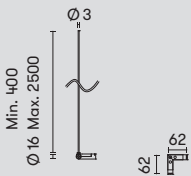
71-8254-05-05 ■ 90° horizontal connector | Conector 90° horizontal | Connecteur 90° horizontal
