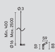
71-8253-05-05 ■ 120° connector | Conector 120° | Connecteur 120°
