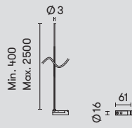
71-8256-05-05 ■ Linear connector with lateral input | Conector lineal con entrada lateral | Connecteur linéaire avec entrée latérale
