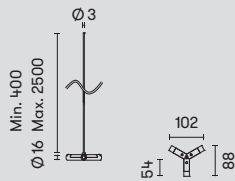
71-8251-05-05 ■ Y connector | Conector Y | Connecteur Y
