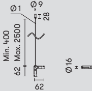
71-8260-05-05 ■ 90° vertical connector | Conector 90° vertical | Connecteur 90° vertical
