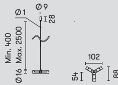
71-8257-05-05 ■ Y connector | Conector Y | Connecteur Y
