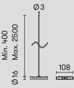
71-8252-05-05 ■ Linear connector with central input | Conector lineal con entrada central | Connecteur linéaire avec entrée centrale
