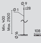
71-8262-05-05 ■ Linear connector | Conector lineal | Connecteur linéaire
