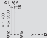
71-8264-05-05 ■ Inter-structure joint fitting | Accesorio de unión entre estructuras | Accessoire de raccord entre structures
