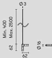
71-8255-05-05 ■ 90° vertical connector | Conector 90° vertical | Connecteur 90° vertical
