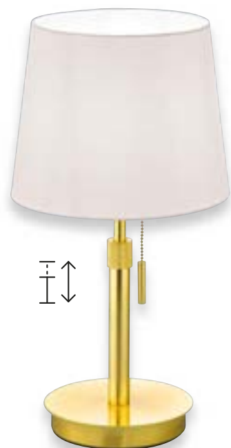
Tischleuchte · Table lamp ↓ 45 – 56 cm, Ø 25,5 cm excl. 1 x E27, max. 60 W
