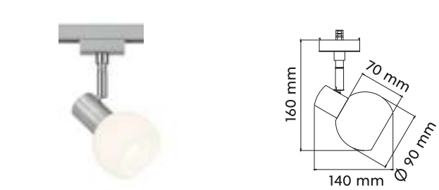
STRAHLER · SPOT excl. 1 x GU10, max. 25 W
