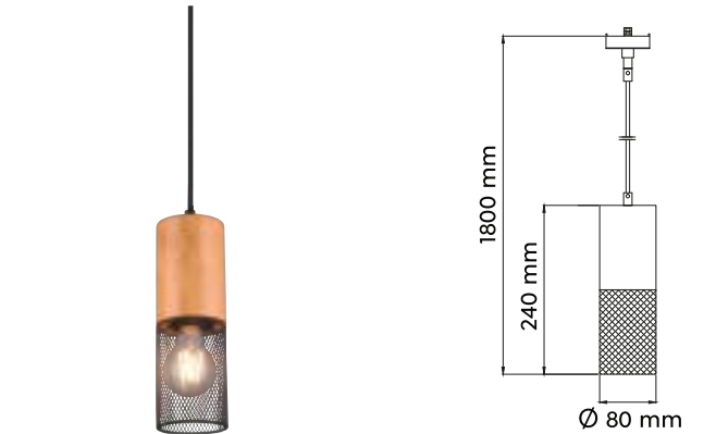
PENDELLEUCHTE · PENDANT excl. 1 x E27, max. 25 W
