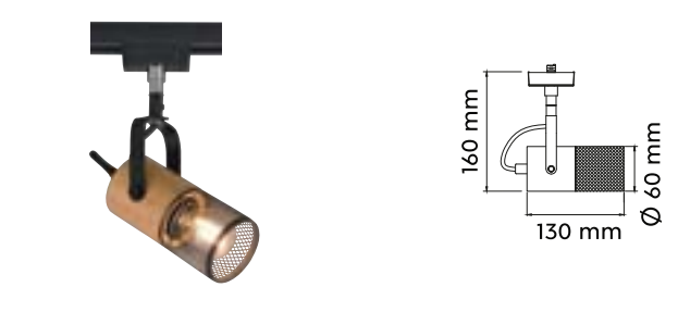
STRAHLER · SPOT excl. 1 x E14, max. 25 W
