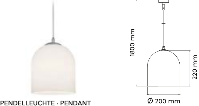
PENDELLEUCHTE · PENDANT excl. 1 x E14, max. 25 W
