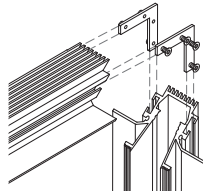
Giunzione grande angolo Large corner junction
